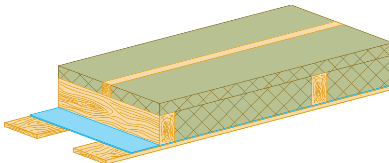
Рис. 3.3. Правильно уложенная теплоизоляция
